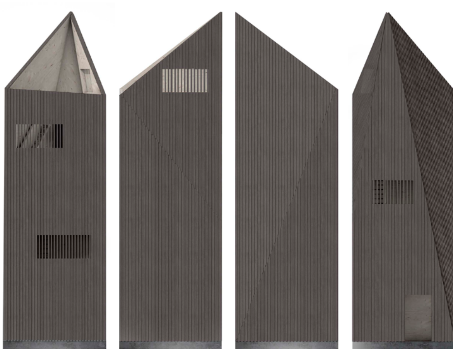
Köykkyrin näkötorni julkisivut 1:100
