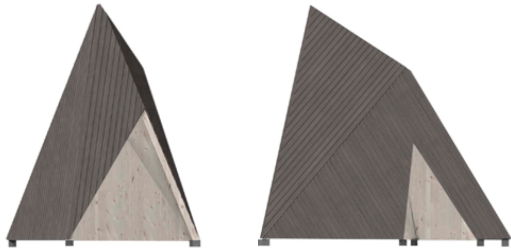
Köykkyrin laavu julkisivut 1:100
