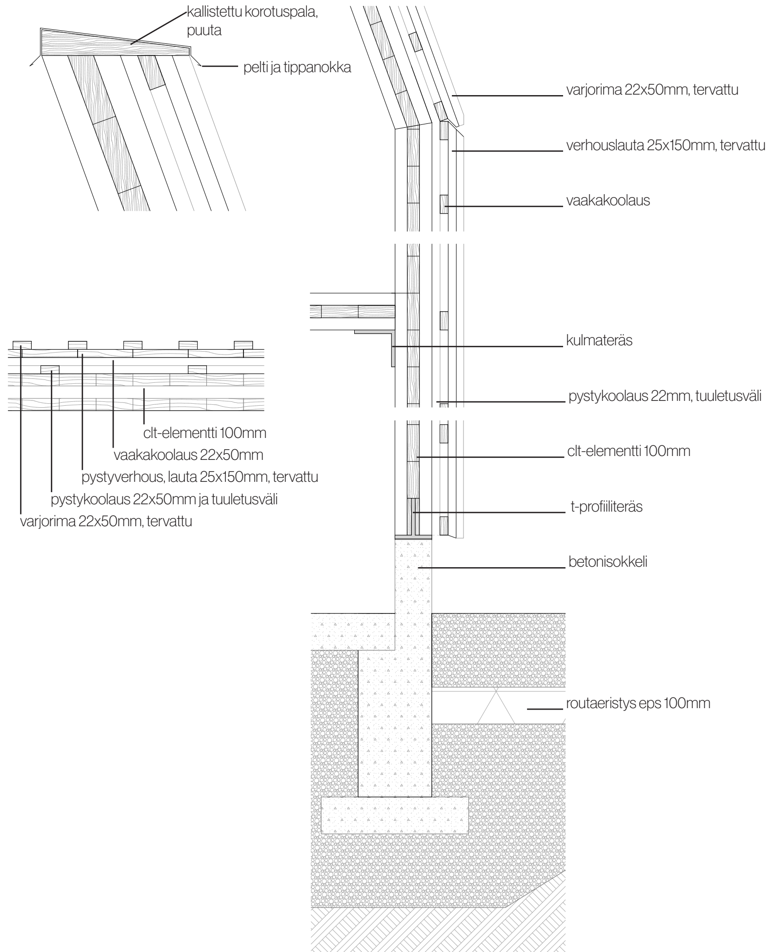
rakenneleikkaukset 1:10/5
