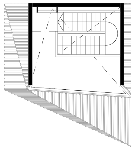
pohjakerros
