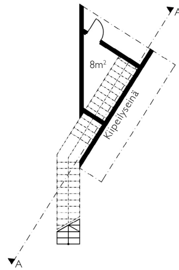
Pohjapiirros 1m 1/200
