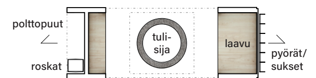
pohja 1:100
