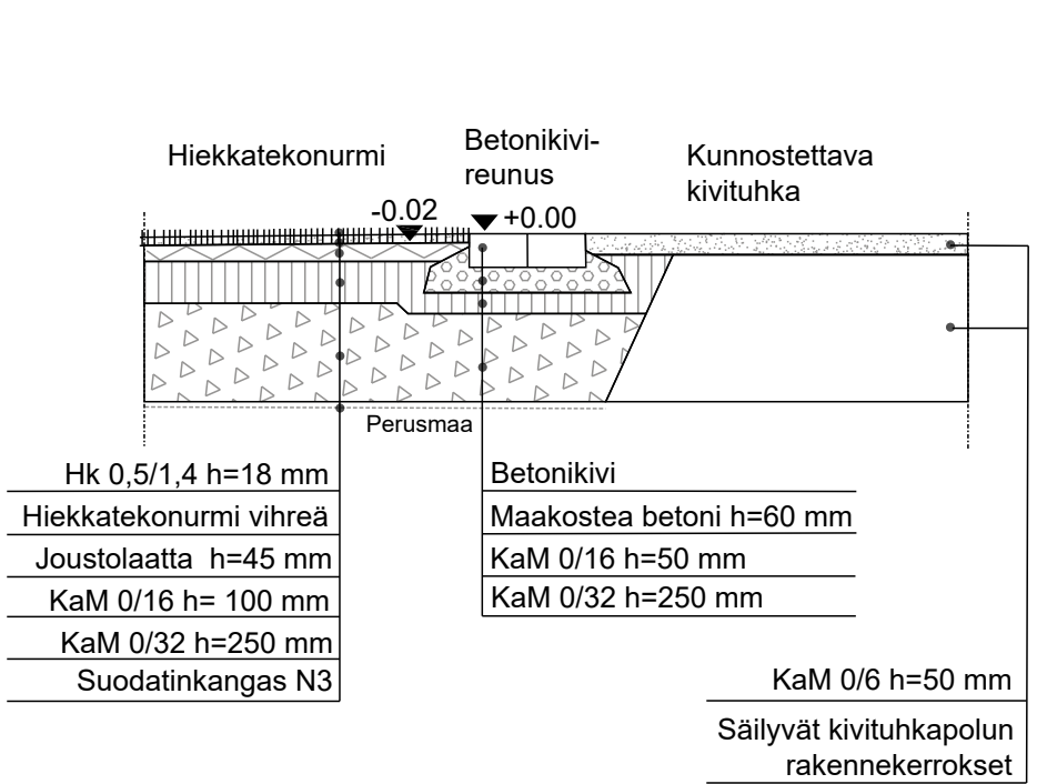
LEIKKAUS B-B Hiekkatekonurmen betonikivireunuksen asennus 1:20
