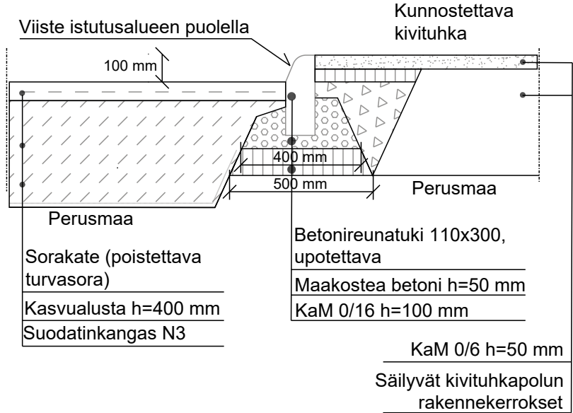
LEIKKAUS A-A Upotettavan reunakiven asennus 1:20
