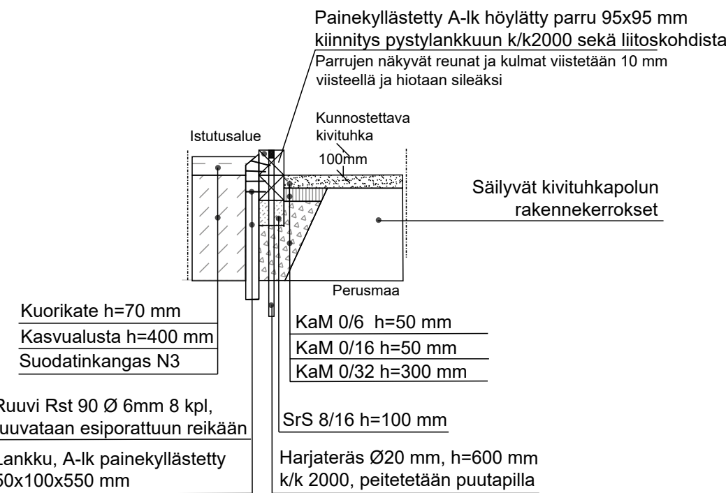
LEIKKAUS C-C Vaakaparruneunus 1:20
