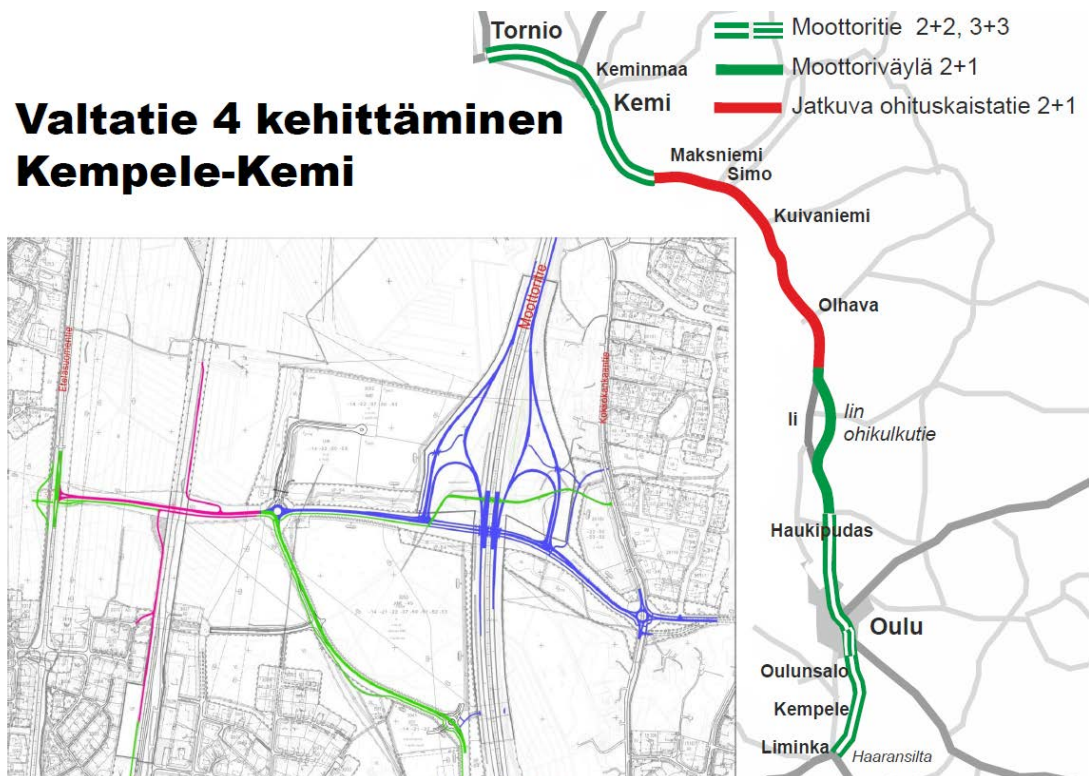
Valtatie 4, Zateeliitin alueen eritasoliittymän toteutuksen vaiheistus.
