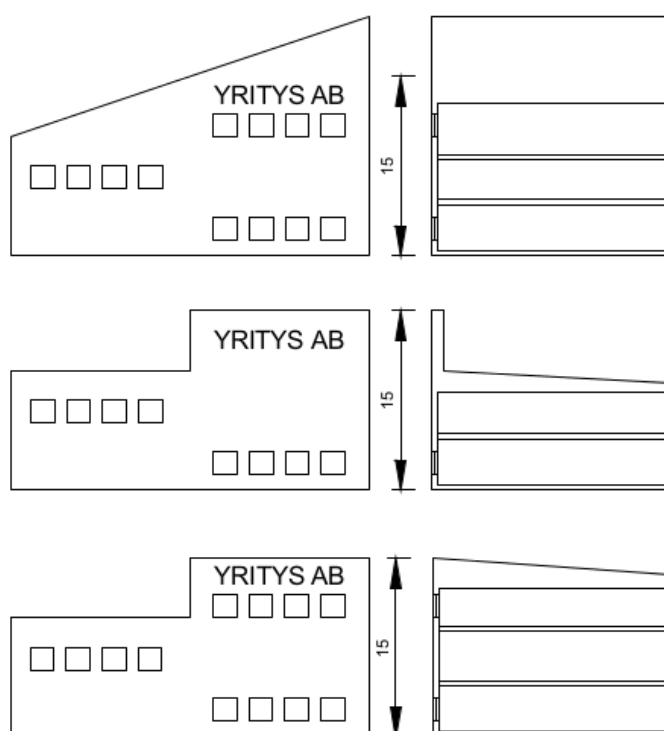
Kuva 2. Esimerkkejä rakennuksen massoittelevuudesta, jolla julkisivun haluttu korkeus voidaan saavuttaa.
