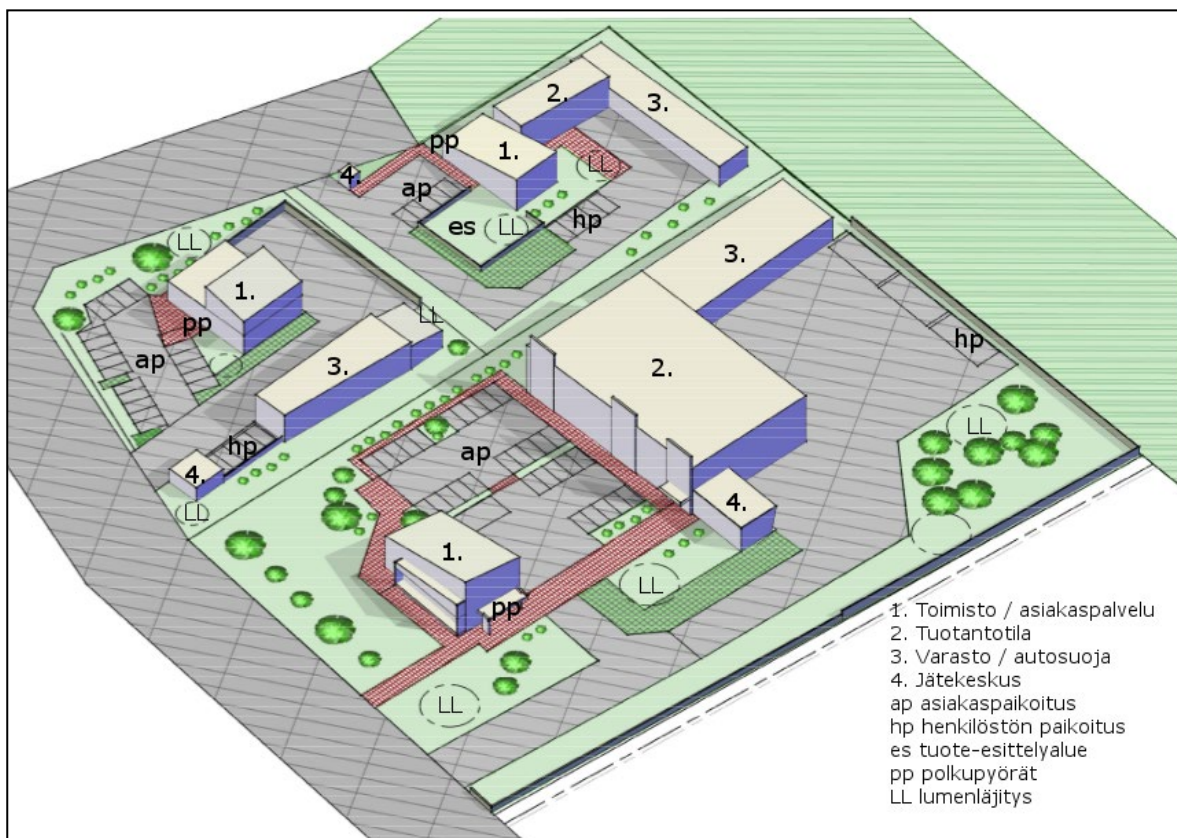
Kuva 1. Esimerkkejä eräiden rakennusten ja toimintojen sijoittelusta yritystonteille.
