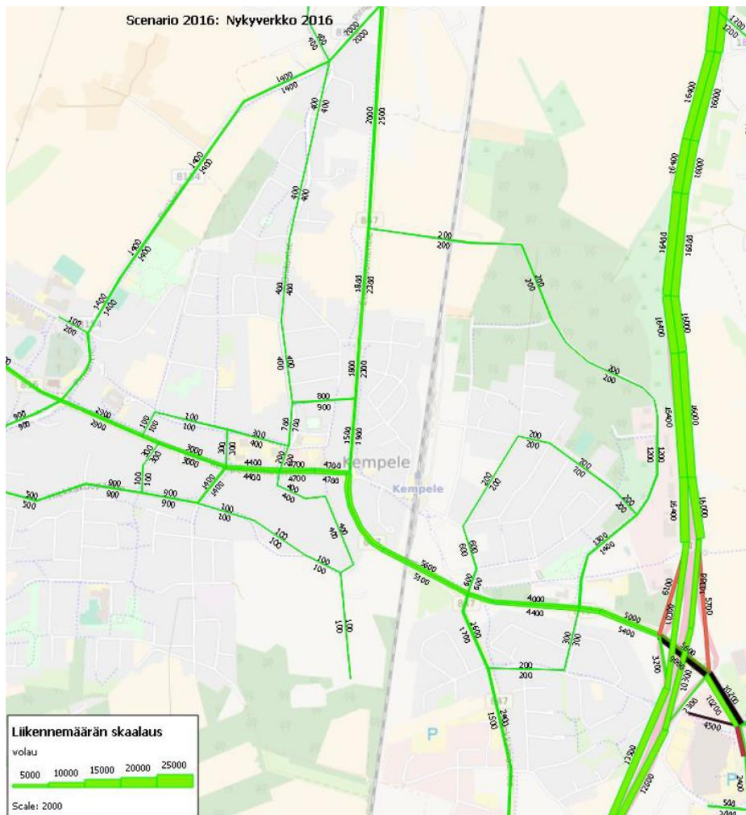
Nykyverkko, nykytilanne: Kempeentien liikennemäärä keskustassa 9400 vrk ja kasvaisi ennusteen mukaan 12.000 ajoneuvoon vuonna 2040 (Ramboll 2016)
