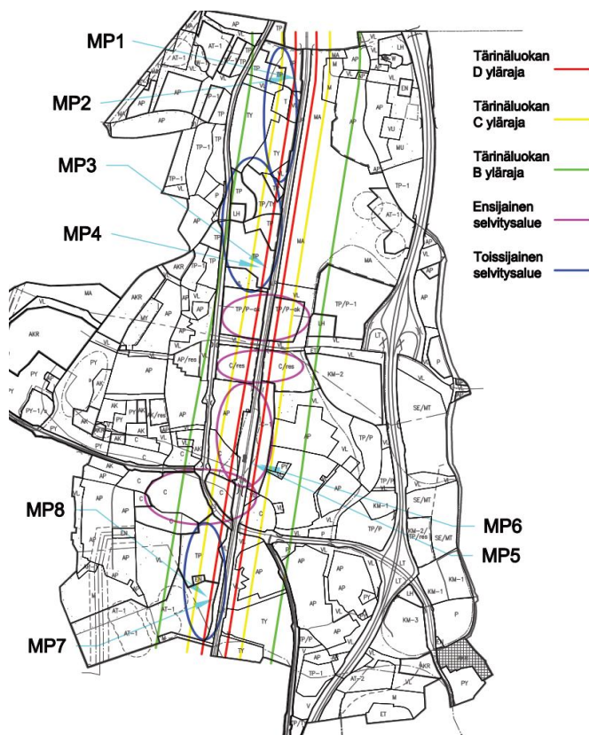
Tärinäselvityksen tärinäluokkien rajat suhteessa luonnosvaiheen kaavamerkintöihin.
