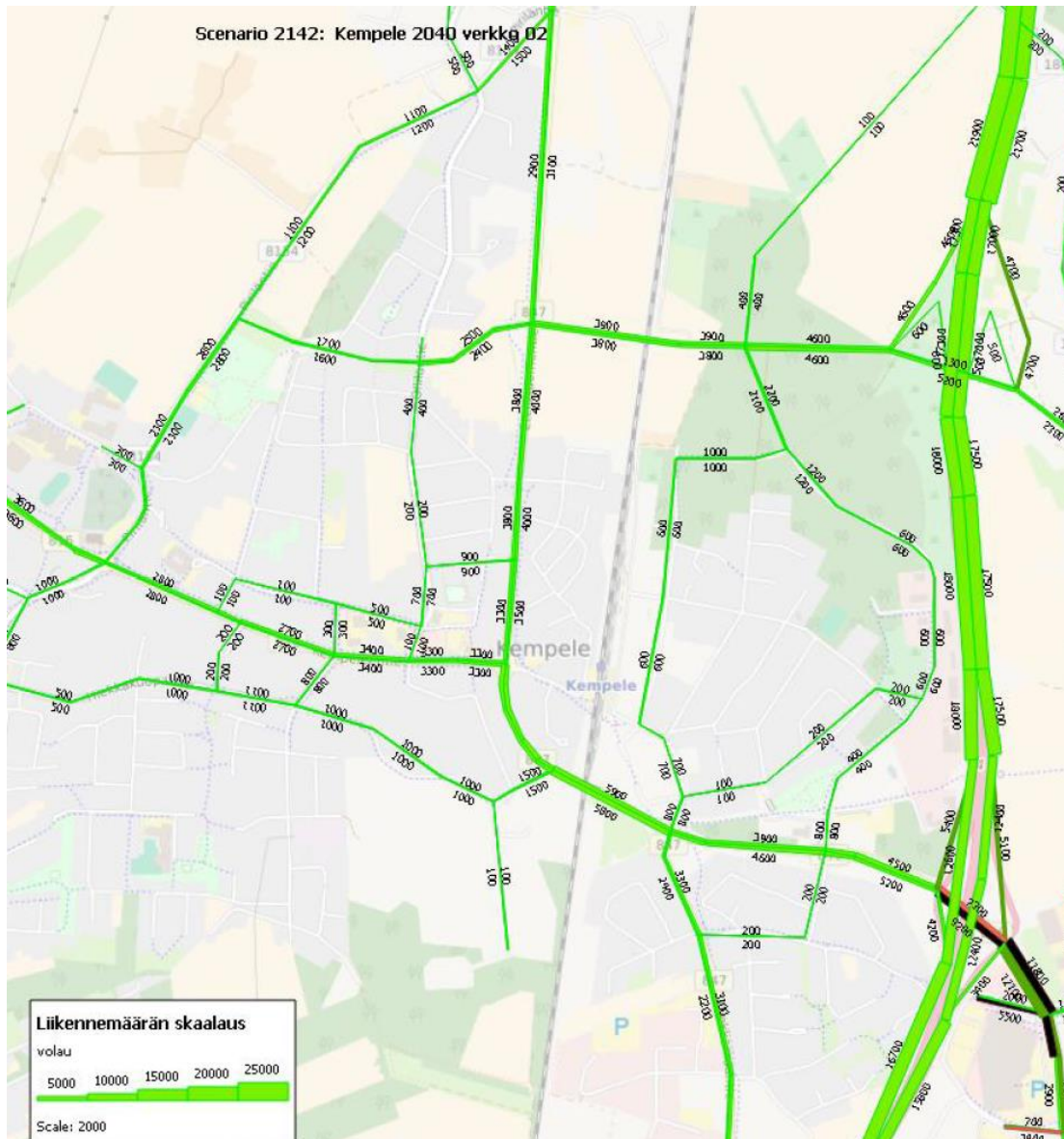
Ennuste 2040, poikkirsi Piriläntielle asti: Kempeleentien liikennemäärä keskustassa 6600 ja poikkiorrella 3300 ajoneuvoa vuorokaudessa (Ramboll 2016)
