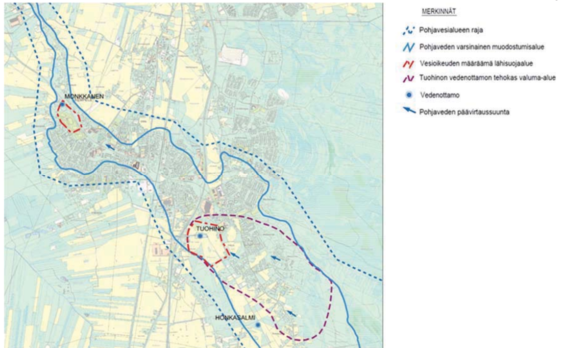
Kuva 9. Kempeleen kunnan alueella sijaitsevien vedenottamoiden sijainnit, Monkkasen ja Tuohinon vedenottamoiden lähisuoja-alueet sekä Tuohinon vedenottamon tehokas valuma-alue. (Pöyry Finland Oy 2015)
