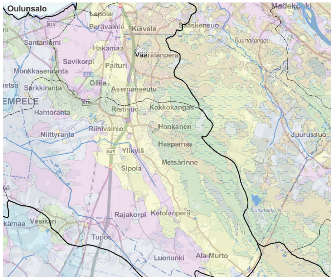
Kuva 1. Kempeleen kunnan alueen maaperäluokitus (MML Paikkatietoikkuna): vihreä = hiekka, keltainen = karkea hiehta, lila = hieno hiehta, vaalean ruskea = hiekkamoreeni. Sinisellä katkoviivalla on merkitty kuntarajat, kapealla mustalla pohjavesialue ja valuma-alue rajat, paksulla mustalla päävaluma-alue rajat.
