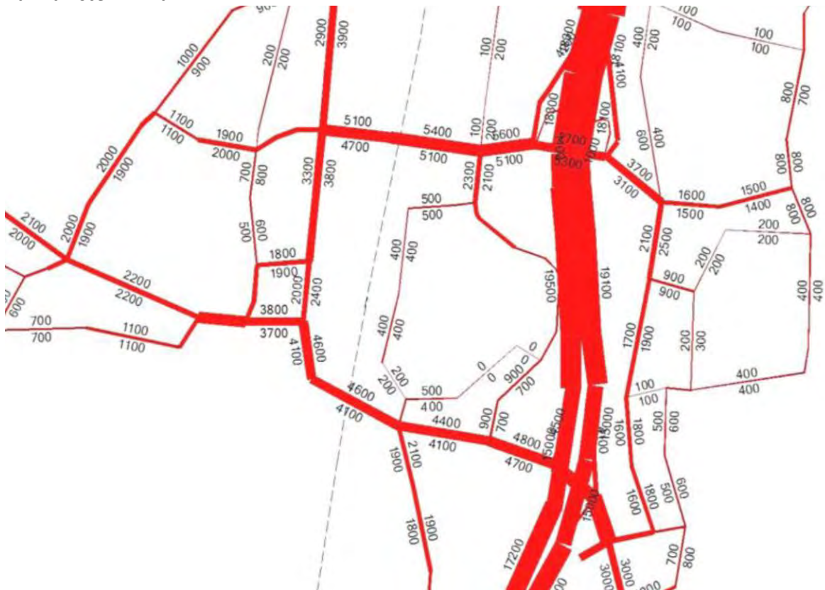
Kuvan tarkastelussa on huomioitu Zatelliitin uusi eritasoliittymä (Kempeleenportti), jolloin uusi poikittaisyhteys vähentää Ketolanperäntien kuormitusta merkittävästi (14 300 ajon/vrk > 8 200 ajon/vrk). Liikennemäärätarkastelu Ramboll Oy.
