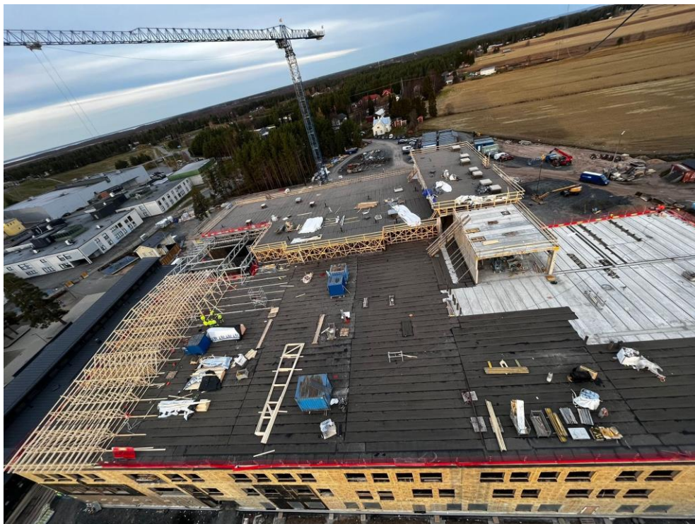
Kuva 2. Työmaatilanne 24.10.2022. Kuvan edustalla C-lohkon runkotyöt pääosin valmistuneet ja vesikattotyöt aloitettu. B-lohkolla asennetaan teräsrakenne kattoa ja 4.krs IVKH katolle asennettu valmistuneelle osalle pohjahuopa.
